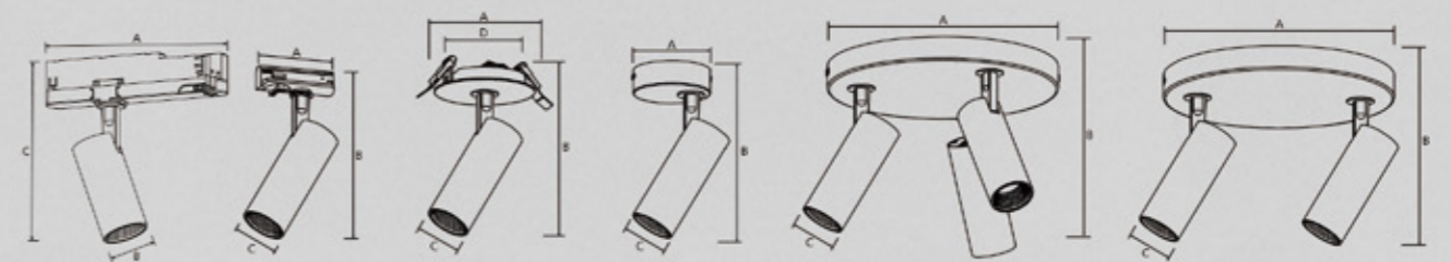
TL62 TL62B TL62C TL62D-8W TL62D-24W TL62D-16W
